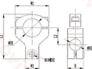
产品关键尺寸图
