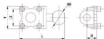
产品关键尺寸图
