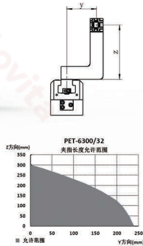
夹指长度允许范围
