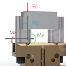
垂直方向最大静载荷
