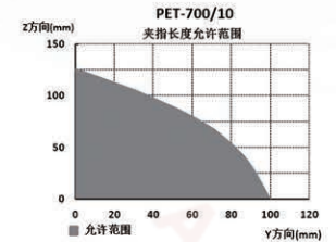
夹指长度允许范围
