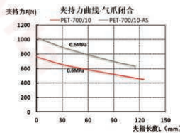
垂直方向最大静载荷
