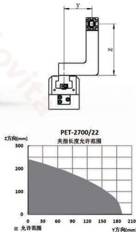
夹指长度允许范围
